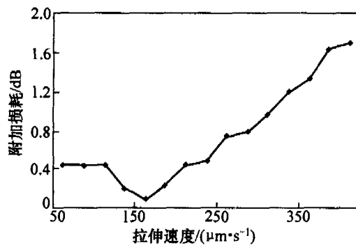
图 6 拉伸速度与附加损耗的关系
