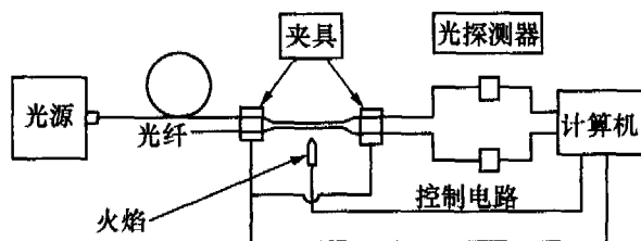
图 3 光纤耦合器实验框图
