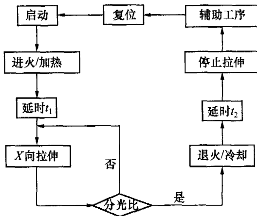
图 4 熔锥型光纤耦合器控制流程
