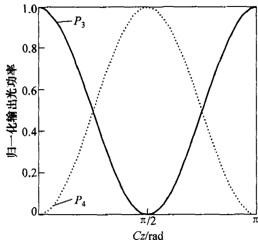
图 2 两输出端的归一化光功率
