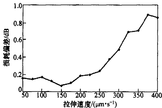
图 7 拉伸速度与损耗偏差的关系
