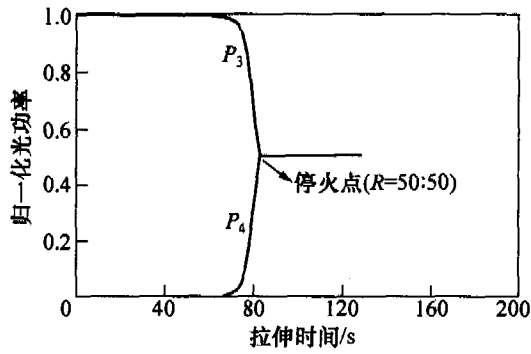
图 5 耦合区归一化光功率分配过程
